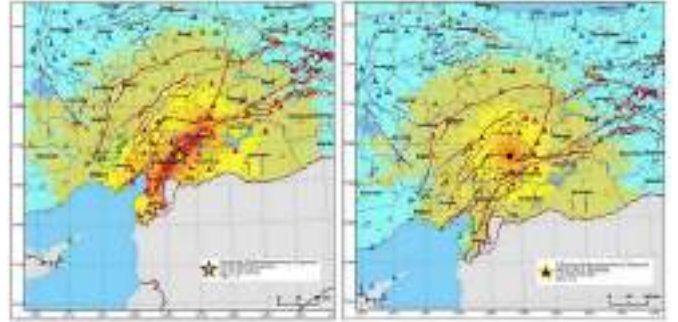
Şekil 2: Kahramanmaraş depremlerinin AFAD-RED tahmini şiddet haritası (06 Şubat 2023 Pazarcık-Kahramanmaraş Mw 7.7, Elbistan-Kahramanmaraş Mw 7.6 Deprem Ön Değerlendirme Raporu, AFAD).
