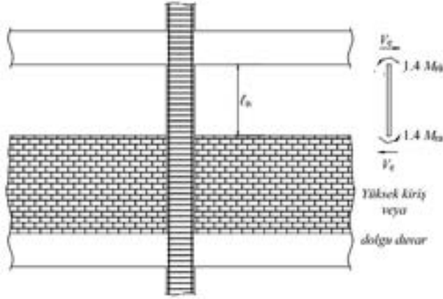
Şekil 4: Dolgu duvarlar ve kolonların tamamen bitişik olması durumunda enine donatıların uygulanması (TBDY-2018, 2018)
