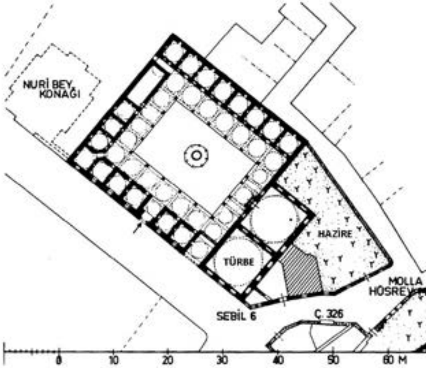
Medresenin Planı. Müller, Bildlexikon, s. 358
